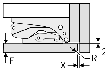
Fig. 100 Монтажний зазор із прилеглою боковиною меблів (F) Товщина фасаду (X) Монтажний зазор, мін. (R) Радіус закруглення фасаду меблів
