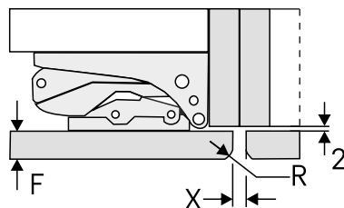
Fig. 101 Монтажний зазор із прилеглими меблевими дверми
