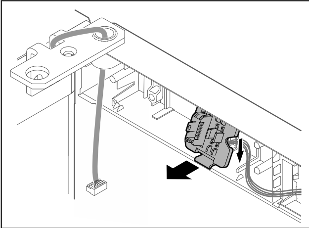
Fig. 22 Кріплення тримача штекера можна повернути на 180°.
