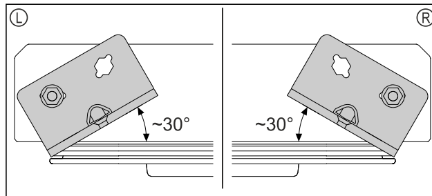
Fig. 45 Дверцята знизу
